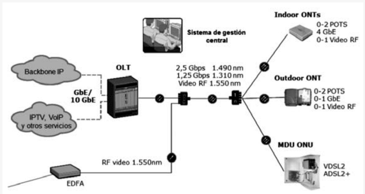
Esquema de una red GPON con posibilidad de transmisión de datos, video y telefonía (de Ramón Millan Tejedor)
