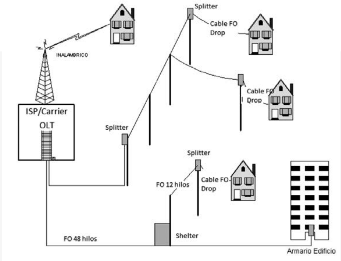
Esquema de instalación de FTTH
